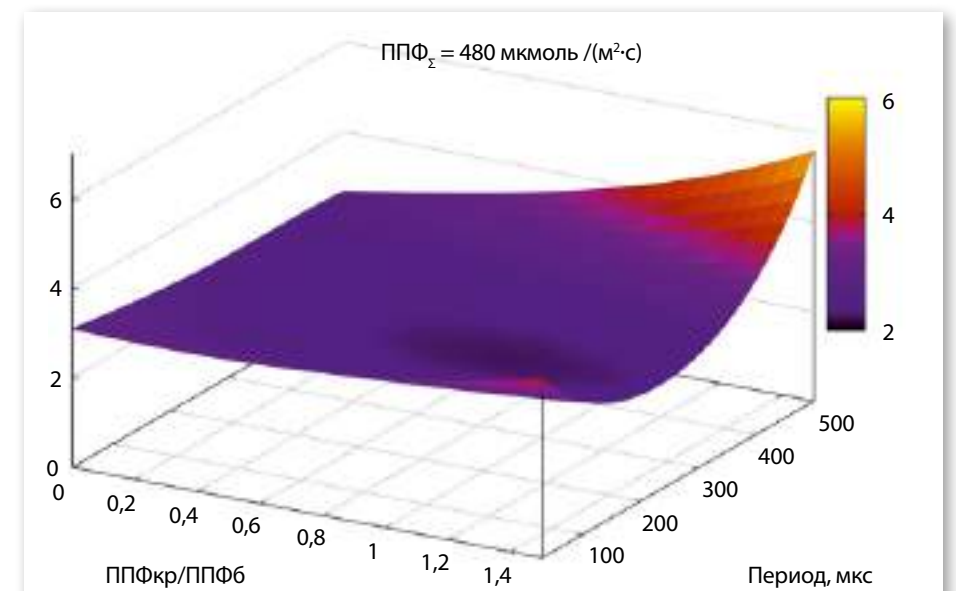
Рис. 3. Трехмерное сечение регрессионной модели критерия оптимальности Q_v
